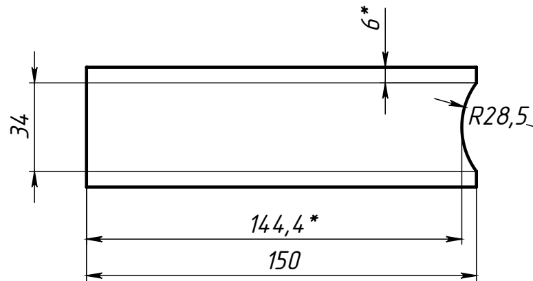
Поз.1 (Основание)
